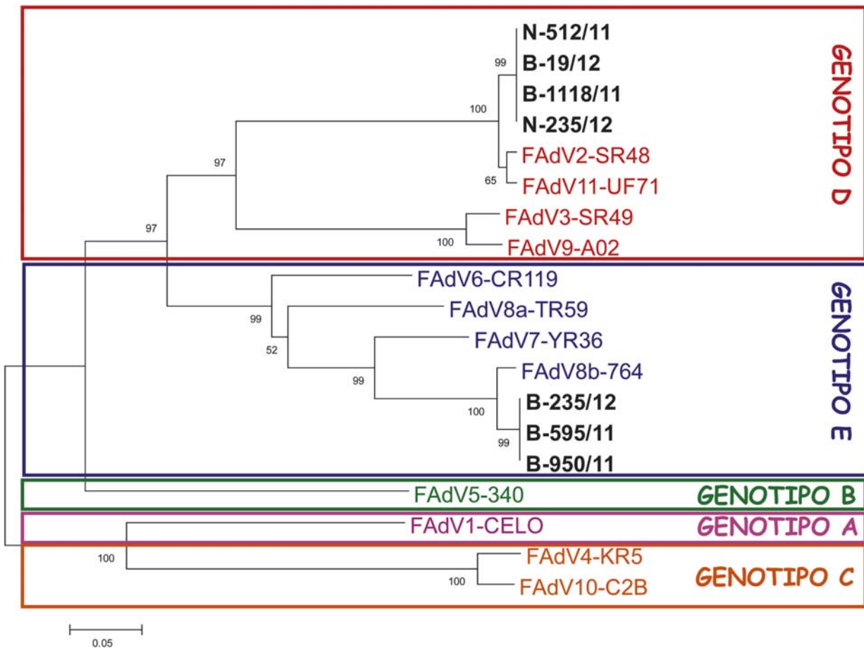
Figura 2. Àrbol filogenètic realitzat a partir de les seqüències nucleotídiques del gen hexon del adenovirus aviar. En negrita els virus involucrats en el brote de IBH en Espanya. En colors, els serotipos de referència pertencents a cada un dels 5 genotipos dels adenovirus.
